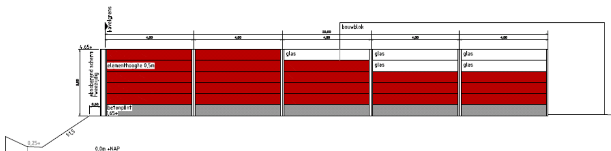
PRINCIPE AANZICHT 1 1:100
